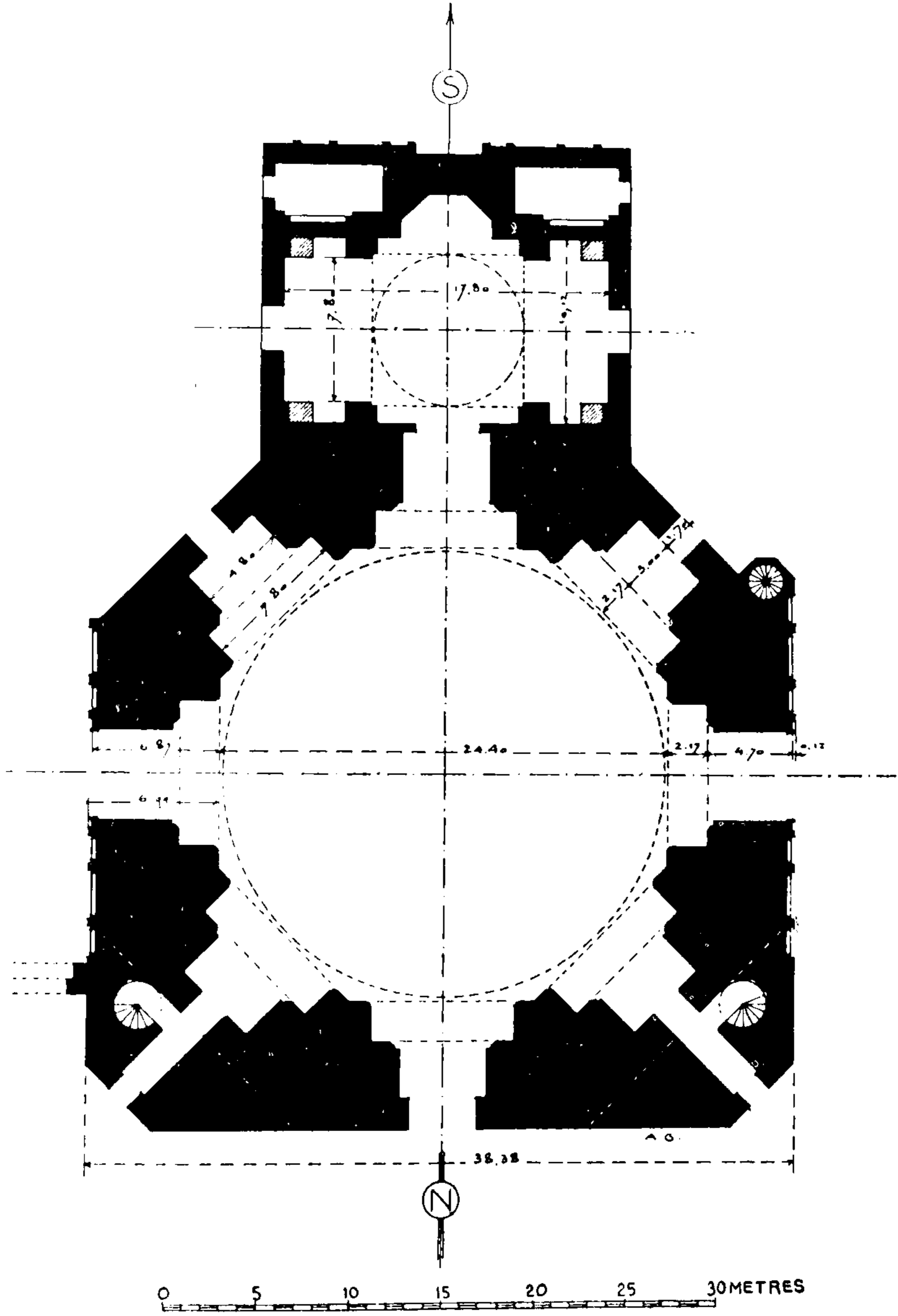
(شكل ٢٨) تخطيط ضريح الهايثو في مدينة سلطانية (عن جودار)
