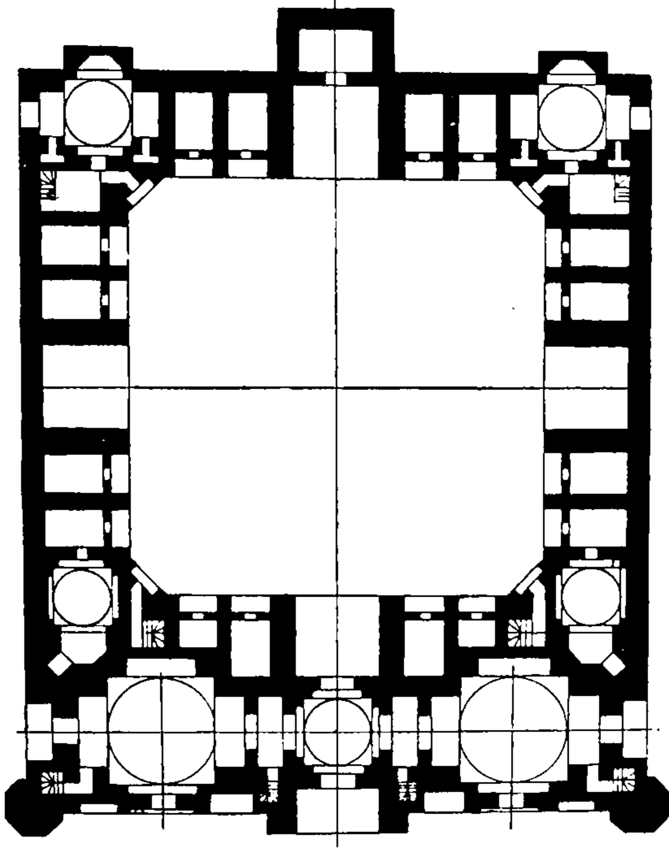
(شكل ٢٩) تخطيط مدرسة خرجرد
